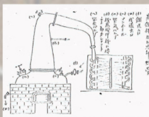
竹鶴レポート・ポットスタイル説明図
